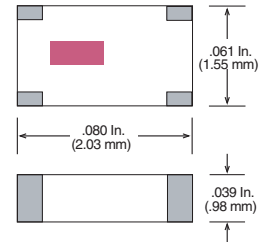
Case 15-4 (EIA 0805 / 1212)
