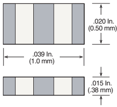
Case 07-1 (EIA 0402/ 1005)
