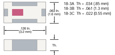
Case 18-3 (EIA 1206 / 3216)
